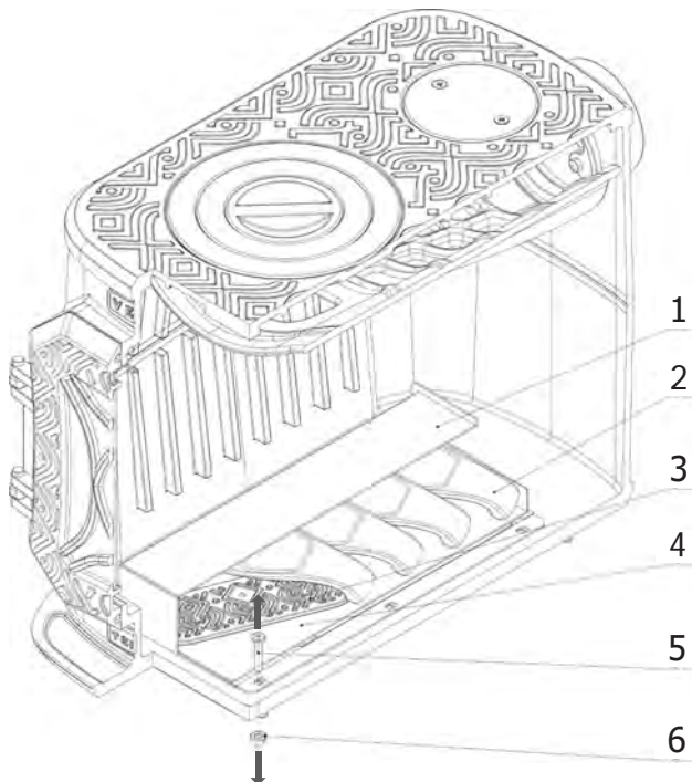
Рисунок 5 — Схема установки ножек на печь
