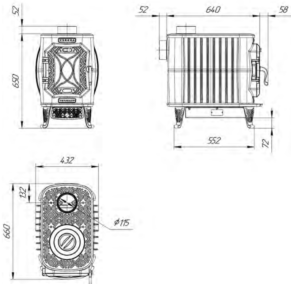
Печь VERONA-200
