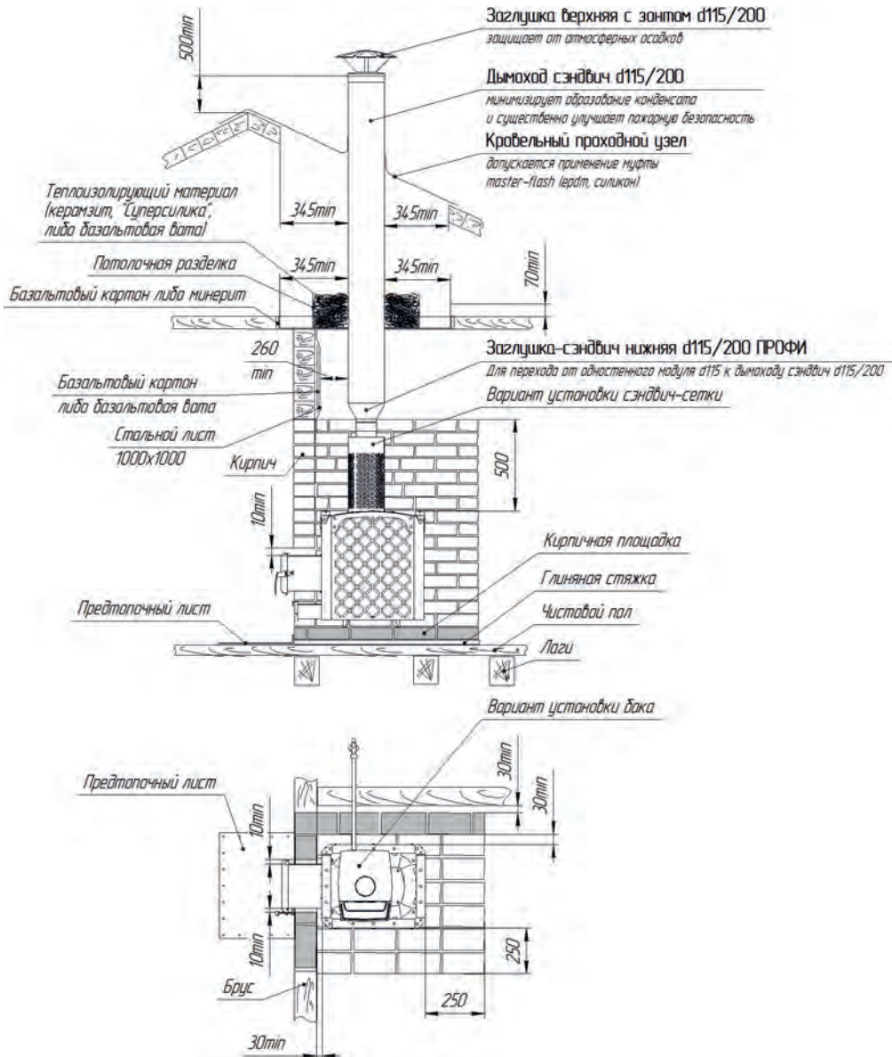
Рисунок 5а - Схема установки печи с кирпичной кладкой
