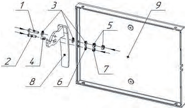
Рисунок 7 — Установка ручки дверки
