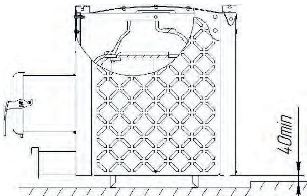
Рисунок 4 — Установка печи «БЫЛИНА» ниже уровня чистового пола
