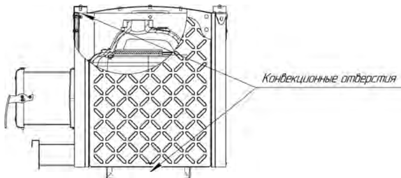
Рисунок 3 — Расположение конвекционных отверстий печи «БЫЛИНА (1.1)»
