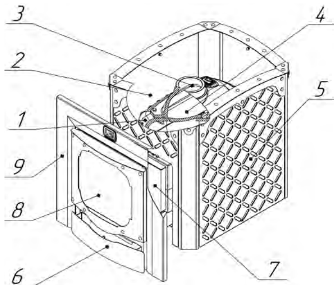
Рисунок 16 - Конструкция печи-каменки «БЫЛИНА Панорама (1.1)»
