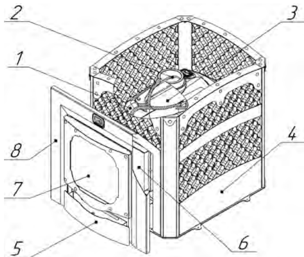
Рисунок 1г - Конструкция печи-каменки «БЫЛИНА-СЕТКА Панорама (1.1)»
