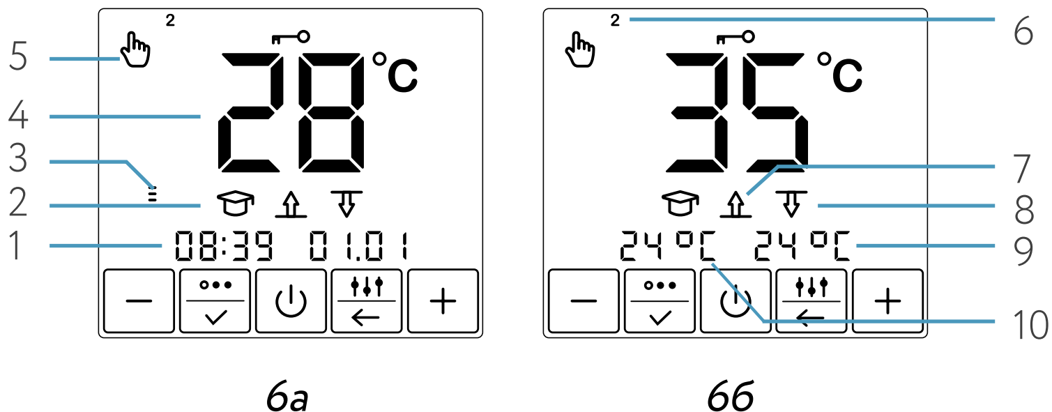
Рис. 6. Основное окно индикации прибора
