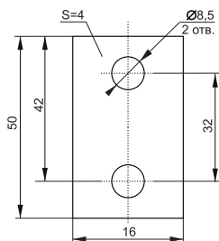
Рисунок 7а – Наконечник переходник для BA88-32M
