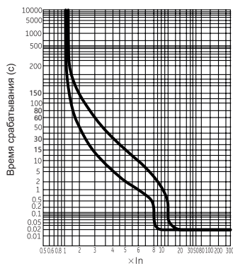
Рисунок 2а - Времятоковые характеристики выключателей BA88-32M с ln 32A
