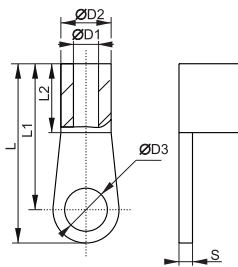
Рисунок 7б – Наконечник переходник для BA88-35M
