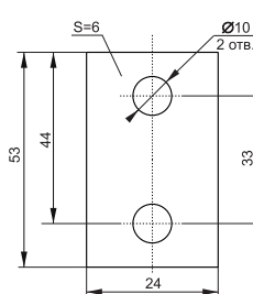
Рисунок 7в – Наконечник переходник для BA88-37M
