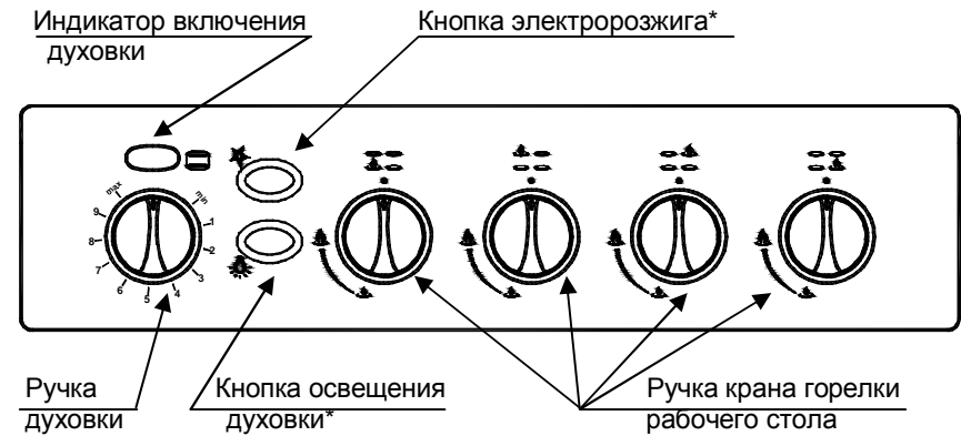
Рисунок 3 – Панель управления плит с электрической духовкой
