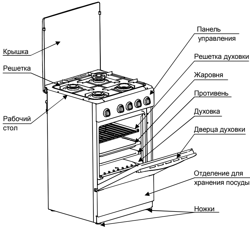
Рисунок 1 – Устройство плиты
