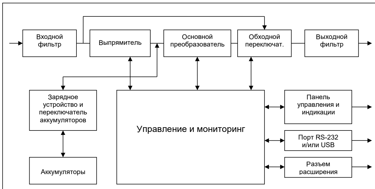
Рис. 1. Блок-схема ИБП
