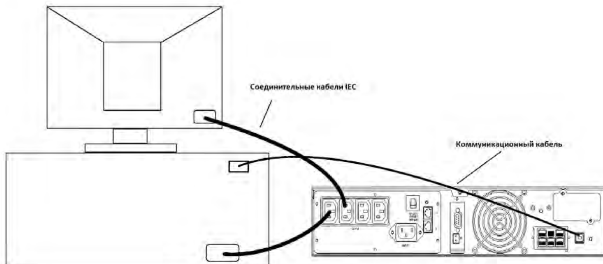
Рис. 3. Пример подключения устройств Plug&Play
