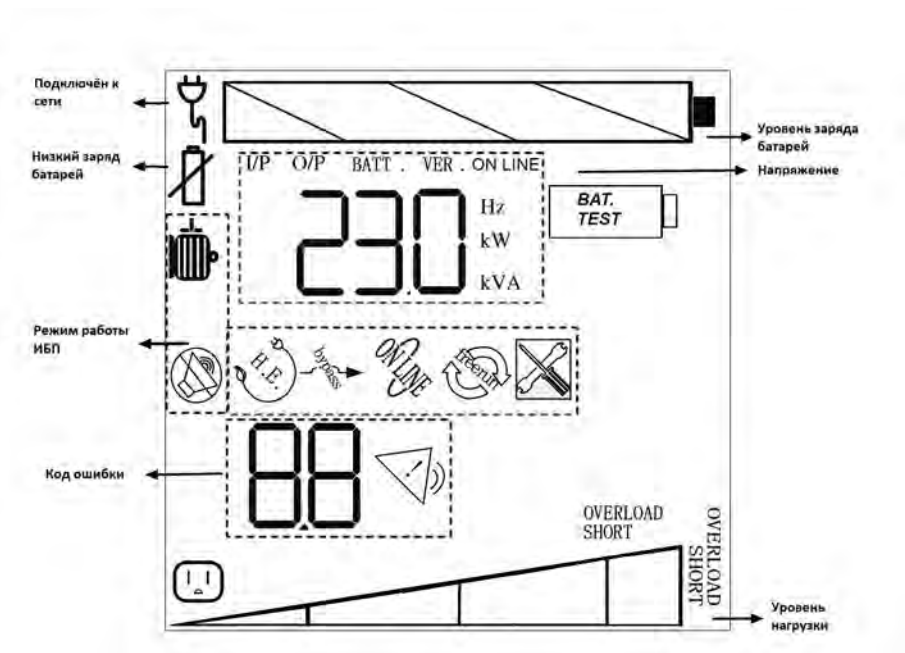
Рис. 7. ЖК-дисплей
