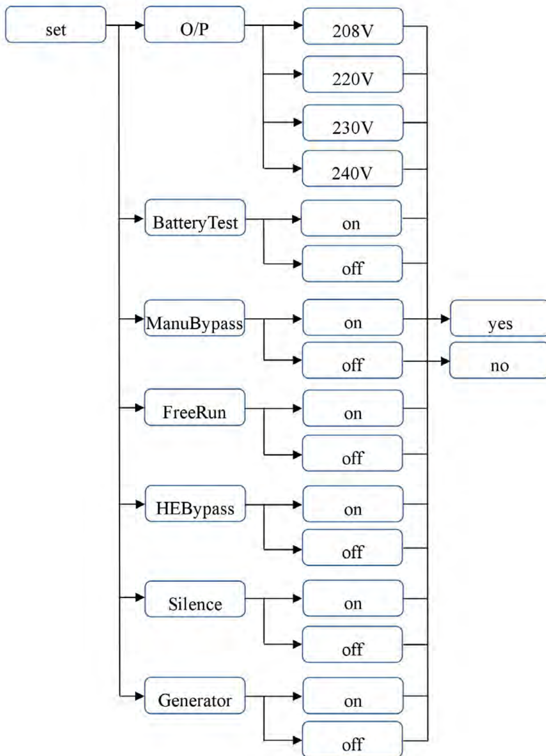
Рис. 9. Настройки ИБП
