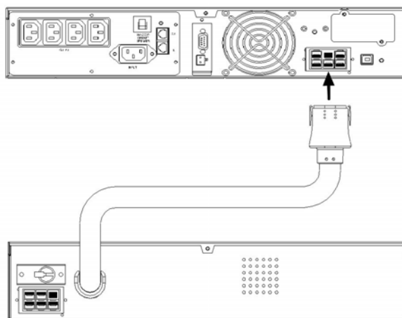
Рис. 4. Подключение внешнего батарейного блока
