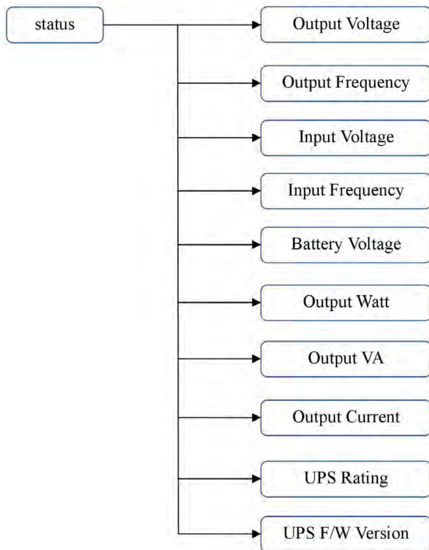
Рис. 8. Состояние ИБП
