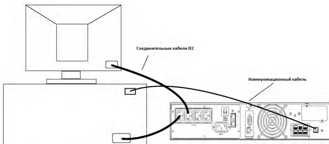
Рис. 5. Пример подключения устройств Plug&Play
