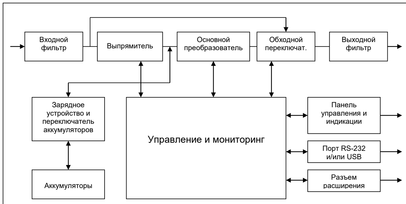
Рис. 7. Блок-схема ИБП
