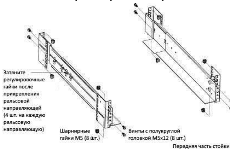
Рис. 2 Закрепление направляющих
