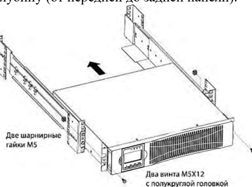
Рис. 4. Монтаж ИБП в стойку.
