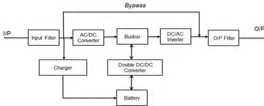
Рис. 1. Блок-схема ИБП
