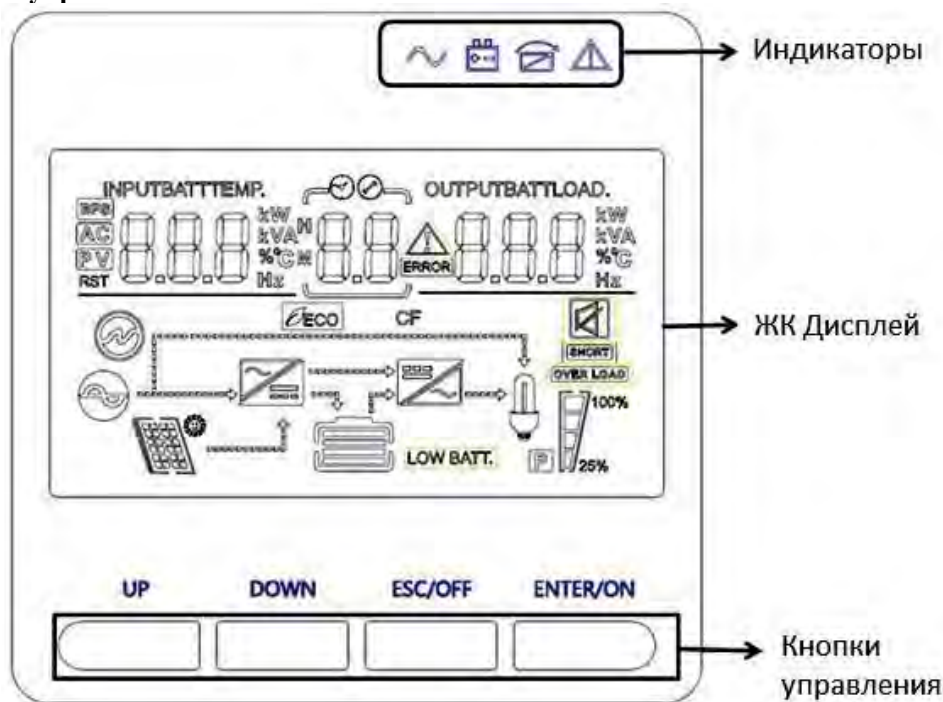
Рис. 2а. Панель управления ИБП
