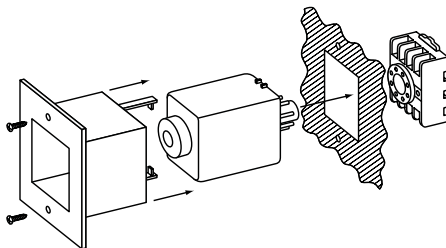
Рисунок 8. Монтаж реле на монтажную плоскость
