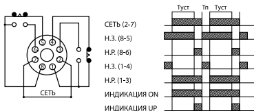
Рисунок 14. Схема работы реле времени PB2, PB3
