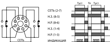
Рисунок 13. Схема работы PB1 (в режиме работы B)
