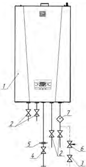
Рис.3. Требования к подключению котла
