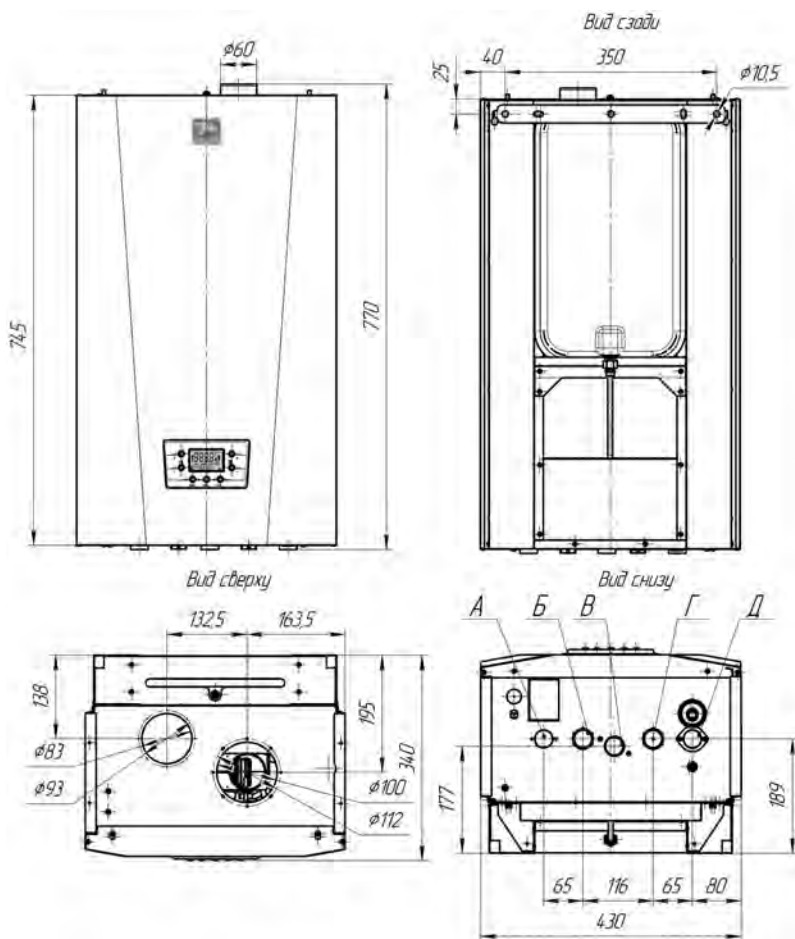
Рис 2.2. Габаритные и присоединительные размеры котлов PRIME-V26,28,32 НО
