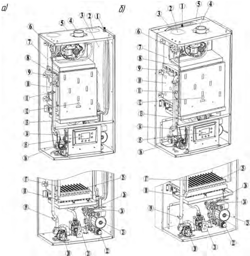
Рис.1. Конструкция котла: а) Prime-V20, 24 HO; б) Prime-V26, 28, 32 HO
