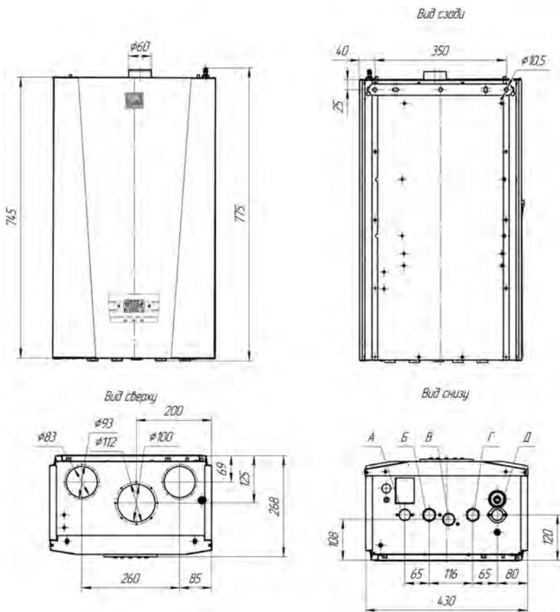
Рис 2.1. Габаритные и присоединительные размеры котлов PRIME-V20,24 NO
