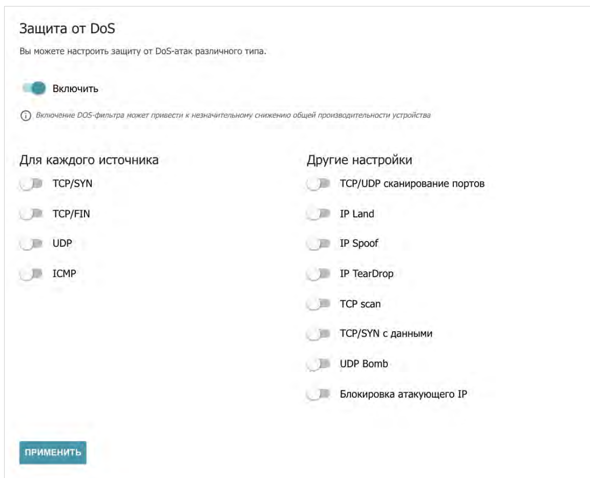
Рисунок 96. Страница Функции / Межсетевой экран / Защита от DoS .
