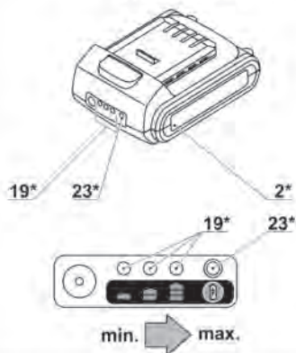
CT21056L-2
