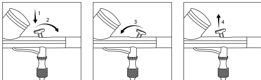
Рис. 4. Аэрограф двойного независимого действия
