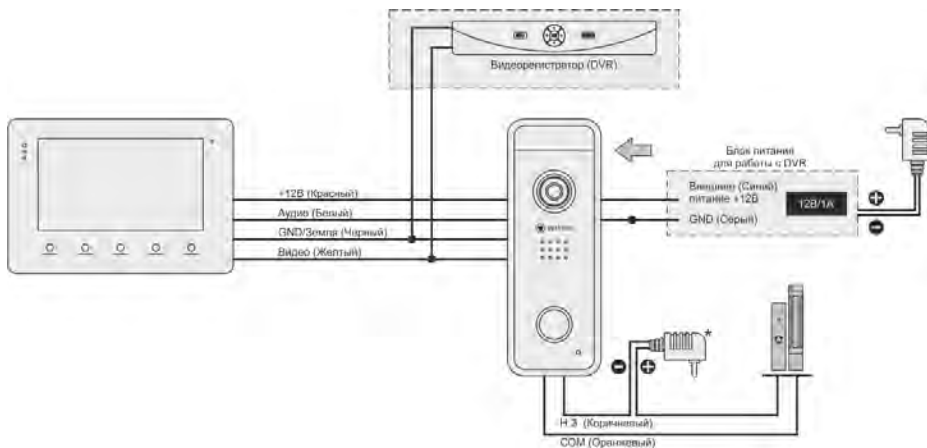
Рисунок 3.Схема подключения №3
