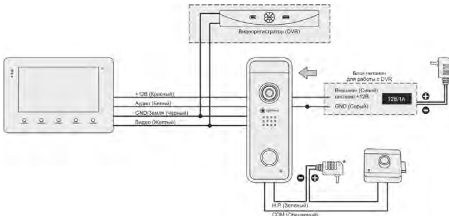
Рисунок 2. Схема подключения №2
