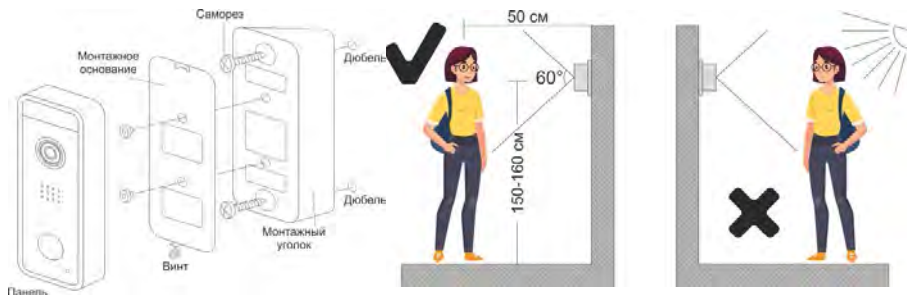
Рисунок 4. Схема установки панели
