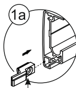
Фиксатор стекла
