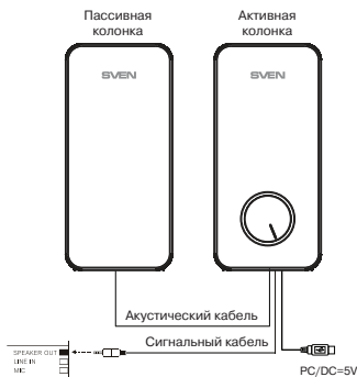
Рис. 2. Схема подключения
