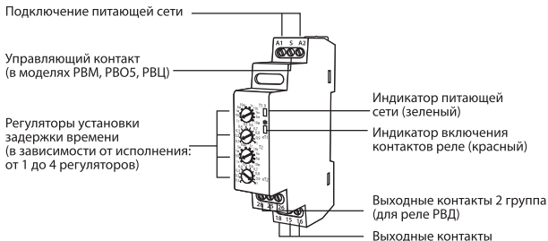
Рисунок 3. Лицевая панель реле
