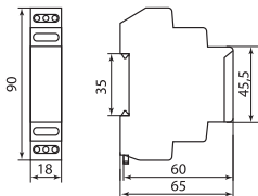
Рисунок 1. Габаритные и установочные размеры реле, мм
