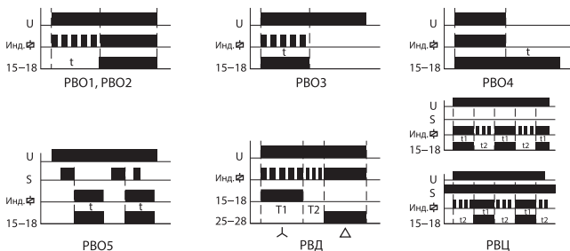
Рисунок 4. Схемы работы реле PBD, PBO1 – PBO5, PBC
