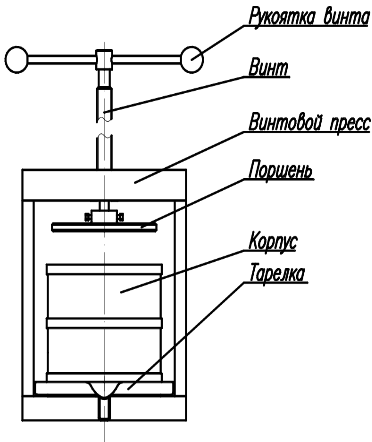
Рис. 1 Устройство изделия
