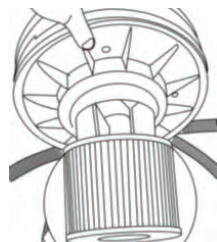
Установка фильтра HEPA (сухая уборка)
