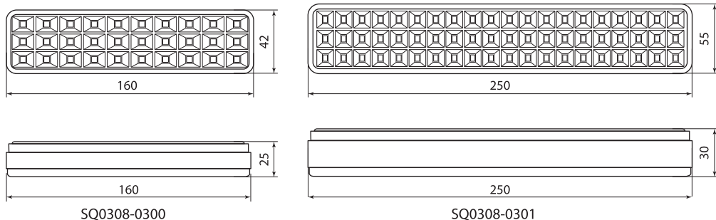
Рисунок 1. Габаритные размеры светильников, мм
