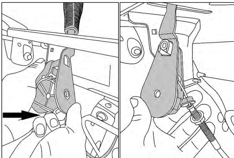
Рис. 22. Установка кронштейна
