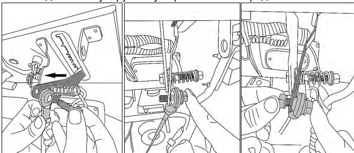
Рис. 14. Установка тяги
