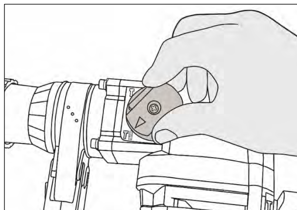
Рис. 11. Переключатель 2
