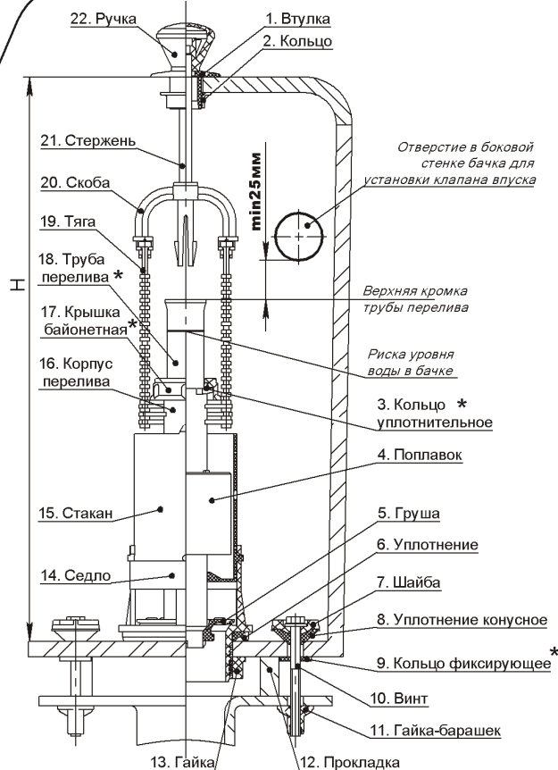
Рис. 2 - Клапан выпуска
