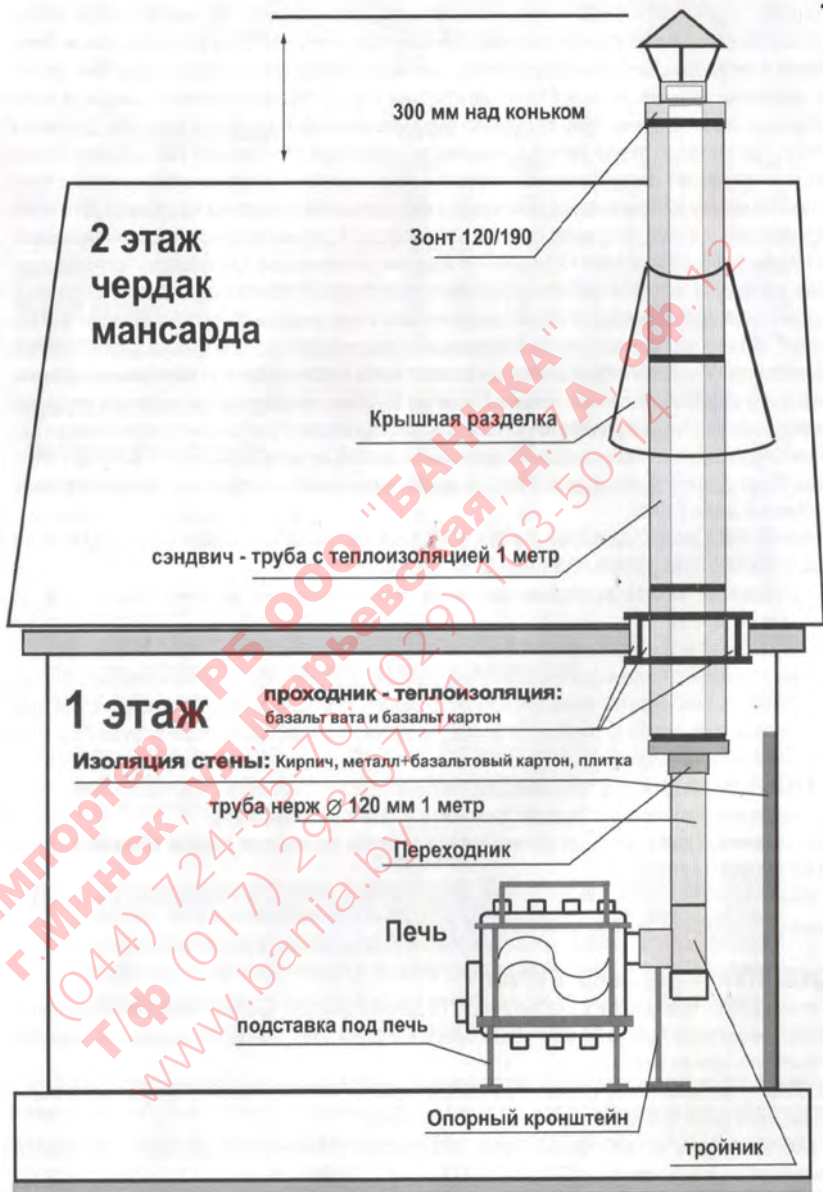
Рис. 2 УСТАНОВКА ПЕЧИ С МЕТАЛЛИЧЕСКИМ ДЫМОХОДОМ (СЭНДВИЧ) ВНУТРИ 2-ЭТАЖНОГО ДОМА
