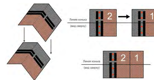
Рис. 33. Устройство рёбер скатов и коньков.
