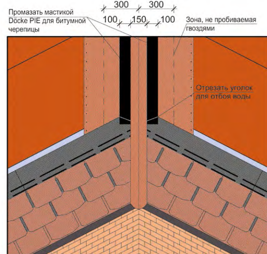
Рис. 27. Выполнение открытой ендовы.
