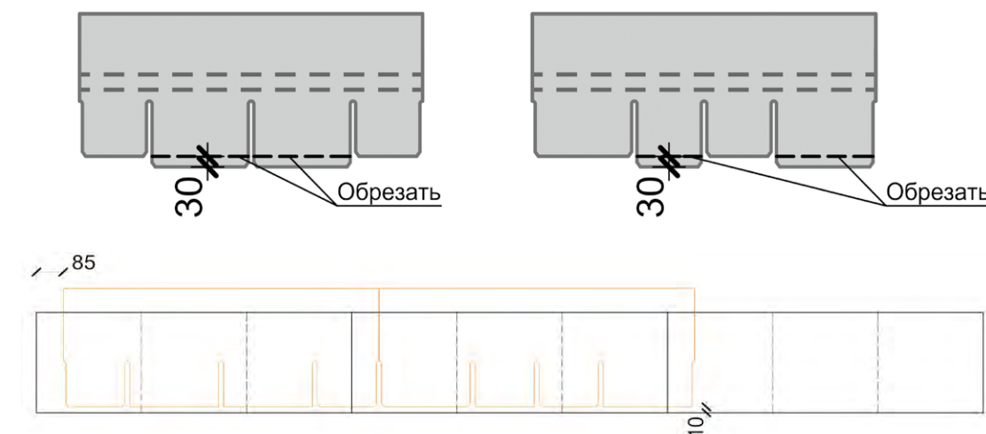
Рис. 23. Подрезка лепестков первого ряда гибкой черепицы коллекции «Саппоро».
