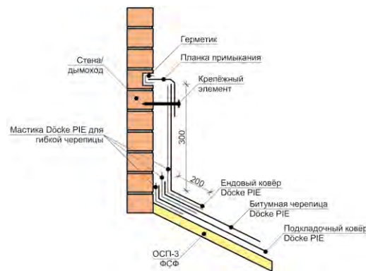
Рис. 31. Примыкание ската крыши к выступающим над ней конструкциям под углом более 90°.
