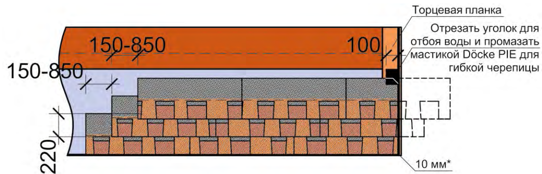
Рис. 25. Схема смещения гонтов по горизонтали и вертикали.
