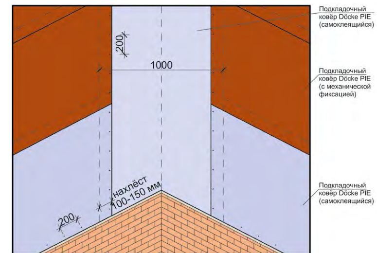
Рис. 12. Схема монтажа подкладочного ковra в ендове и на смежных скатах.
