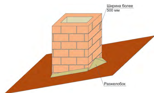
Рис. 30. Примыкание кровли к трубе дымохода шириной более 500 мм.
