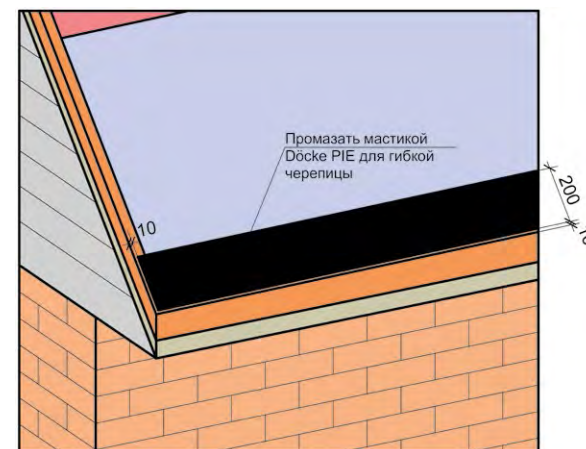
Рис. 22. Герметизация карнизного свеса под укладку ламинированной черепицы Döcke.
