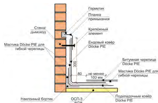
Рис. 32. Примыкание ската крыши к выступающим над ней конструкциям под углом не более 90° включительно.
