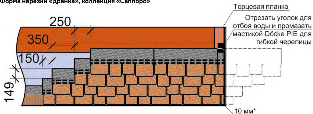
Рис. 26. Схема смещения гонтов по горизонтали и вертикали.
