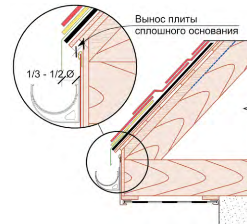
Рис. 6. Устройство выноса первого листа ОСП по отношению к первой доске обрешётки.
