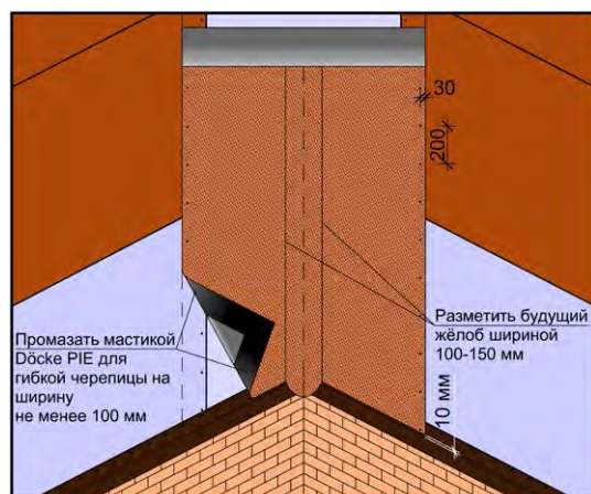
Рис. 14. Монтаж ендового ковра.
