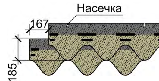
Рис. 24. Схема смещения гонтов по горизонтали и вертикали.
