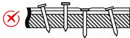
Рис. 3. Пример неправильной забивки гвоздей при монтаже продукции.
