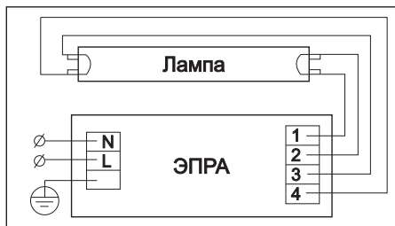
Рис.1 Схема подключения
