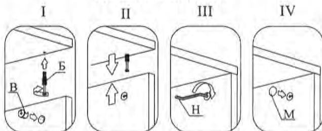
Крепление эксцентриком
