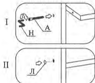
Крепление винтовой стяжкой
