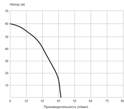
Расходно-напорные характеристики для насосов SN-90/65, 90/90, 90/121, 90/166
