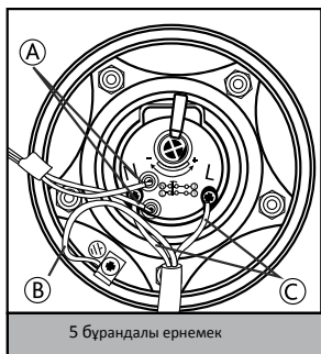
5 бұрандалы ернемек
