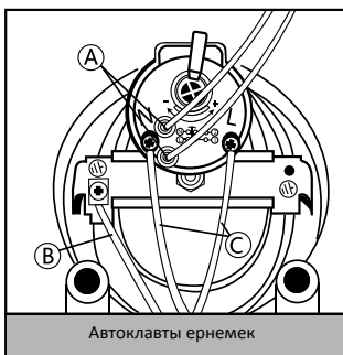
Автоклавы ернемек
