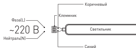
Рис.1. 220В шамчыракты току туташтыруу схемасы
