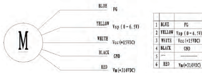
Вентилятор наружного блока (постоянный ток)
