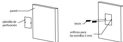
Figura 7-4 Instalación (1)
