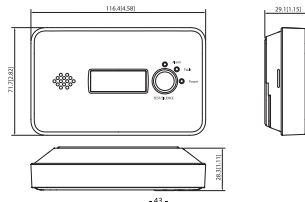
Figura 3-1 Dimensiones (mm[inch])
