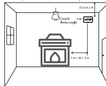
Rysunek 7-2 Instalacja w salonie z urządzeniem spalinywym
