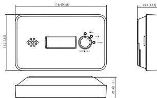
Abbildung 3-1 Abmessungen (mm)
