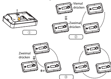
Abbildung 5-1 Gerät verbinden
