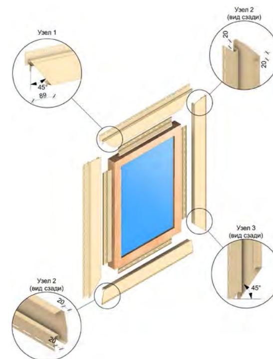
Рис. 9 Обрамление оконного проёма при помощи наличника 89 мм/ 30 мм.
