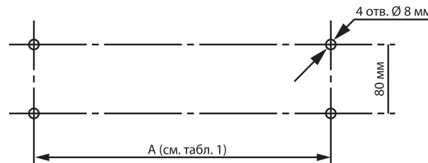
Рис. 1 Схема разметки отверстий
