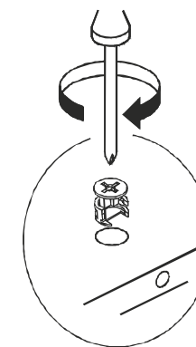
Рис.2 Установка и фиксация стяжки эксцентрика
