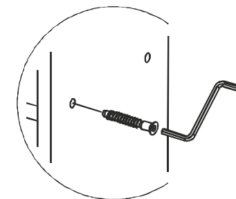
Рис.3 Установка евровинта
