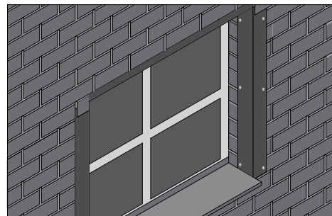
Рис. 8.5. Законченный вид проема
