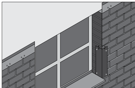
Рис. 8.3. Монтаж оконного наличника сбоку проема
