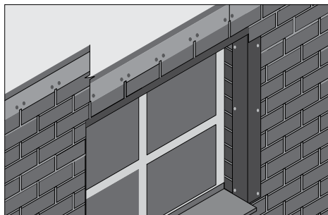
Рис. 8.4. Монтаж оконного наличника сверху проема
