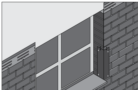
Рис. 8.3. Монтаж оконного наличника сбоку проема
