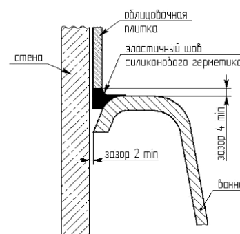
Схема №5. Установка ванны.
