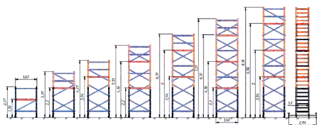
Секция 2 м артикул BT12 1612040
