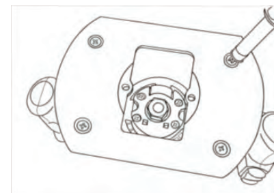
Снятие защитной платформы
