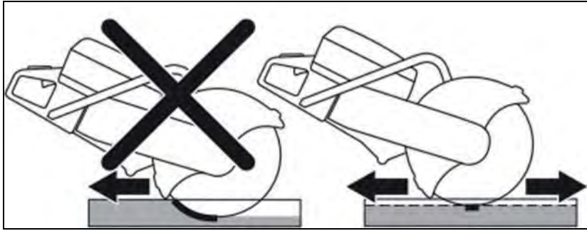
Рис. 19. Эффективная резка
