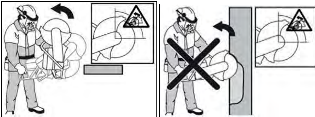
Рис. 20. Возможность отдачи.
