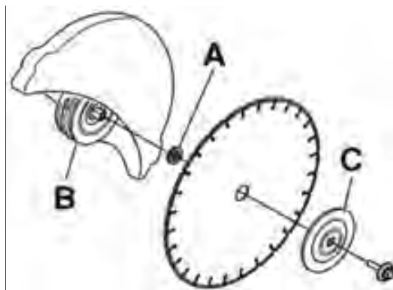
Рис.2 Установка диска
