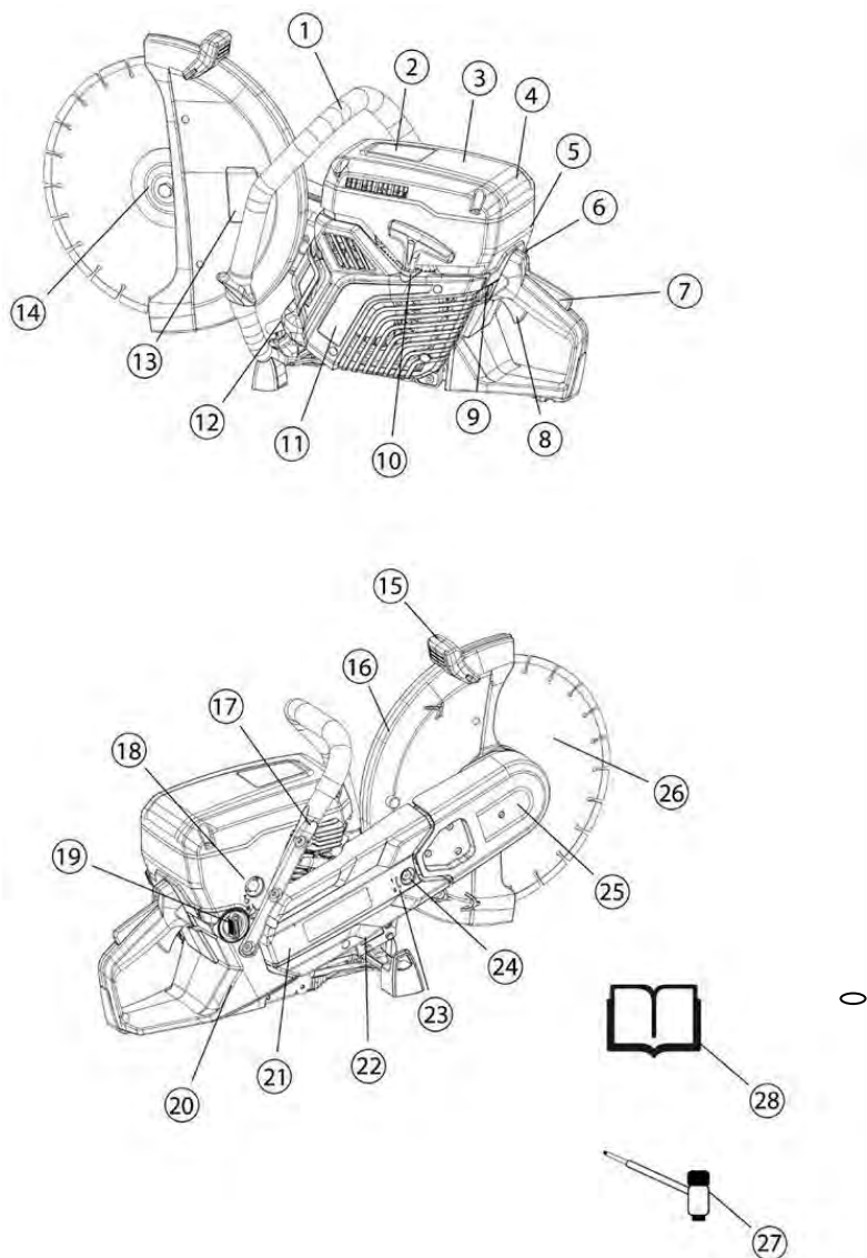
Рис. 1. Общий вид
