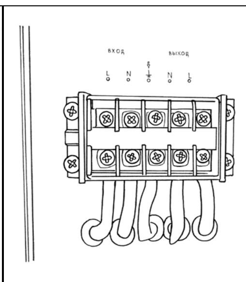
Рис. 7. Схема подключения
