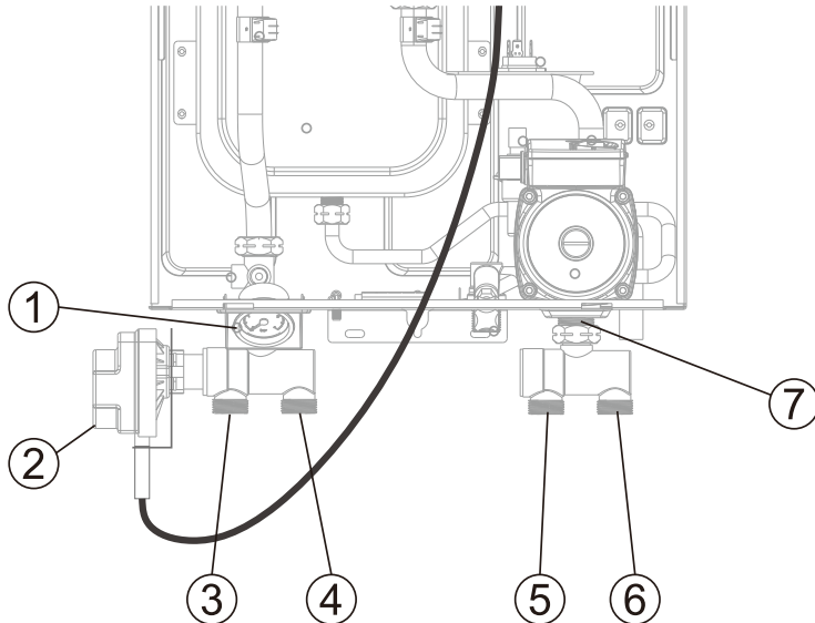
Рис.15. Присоединение трехходового клапана
