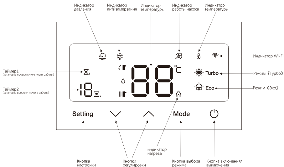
Рис. 3. Панель управления
