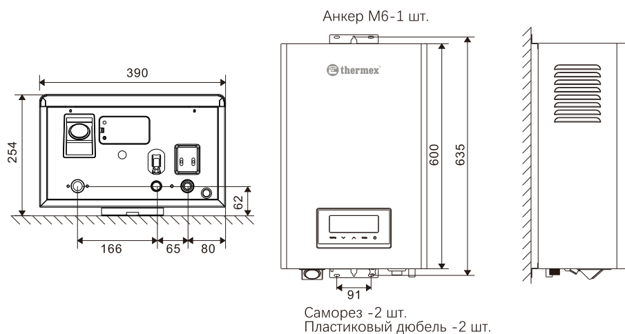
Рис. 6. Монтажные размеры
