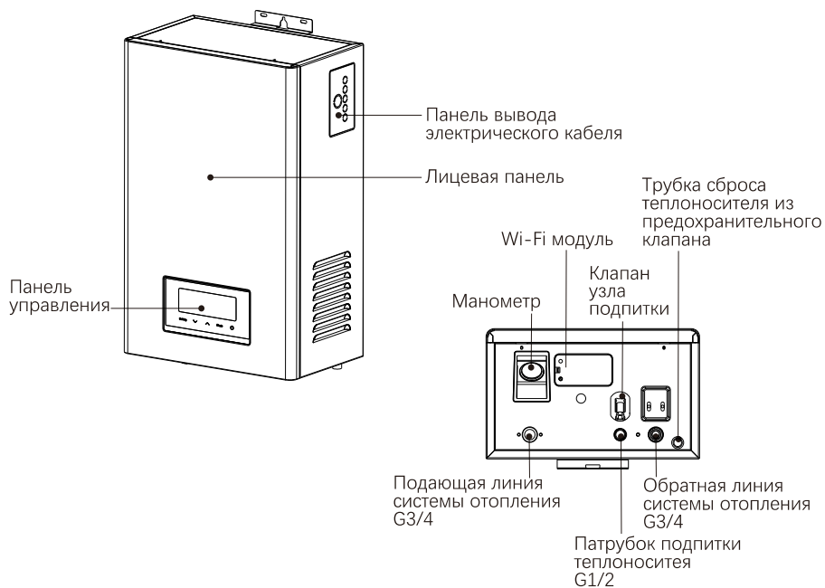
Рис. 1. Конструкция изделия
