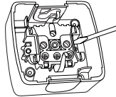
Рисунок 2. Снять механизм розетки, поддев его наколочником плоской отвертки.
