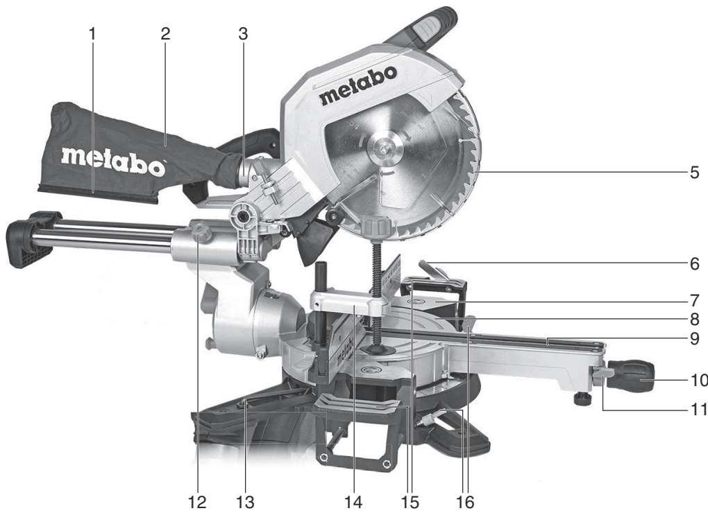
KGS 305 M
