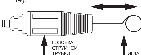
Рис. 14 Чистка форсунки головки струйной трубки
