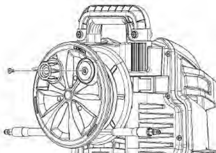
Рис. 2 Установка ручки барабана
