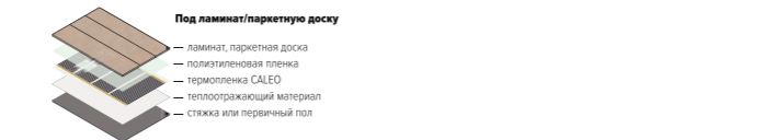
Рис. Схема монтажа теплого пола CALEO под ламинат или паркетную доску
