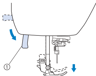
① Рычаг прижимной лапки
