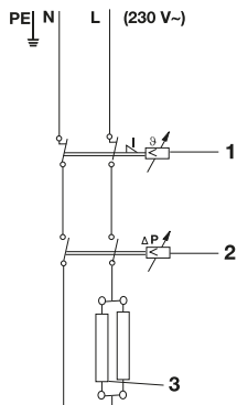
Рис. 6. NP Aquatronic 2.0
