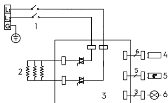
Рис. 6. NPX 8 Aquatronic DIGITAL PRO
