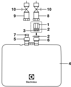
Рис. 1. NP Aquatronic 2.0
